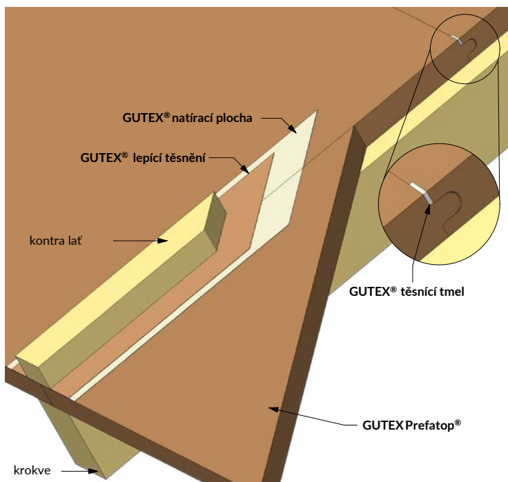
Tupé těsnění pro střešní prvky s GUTEX Prefatop® (detail 1.1.601)
